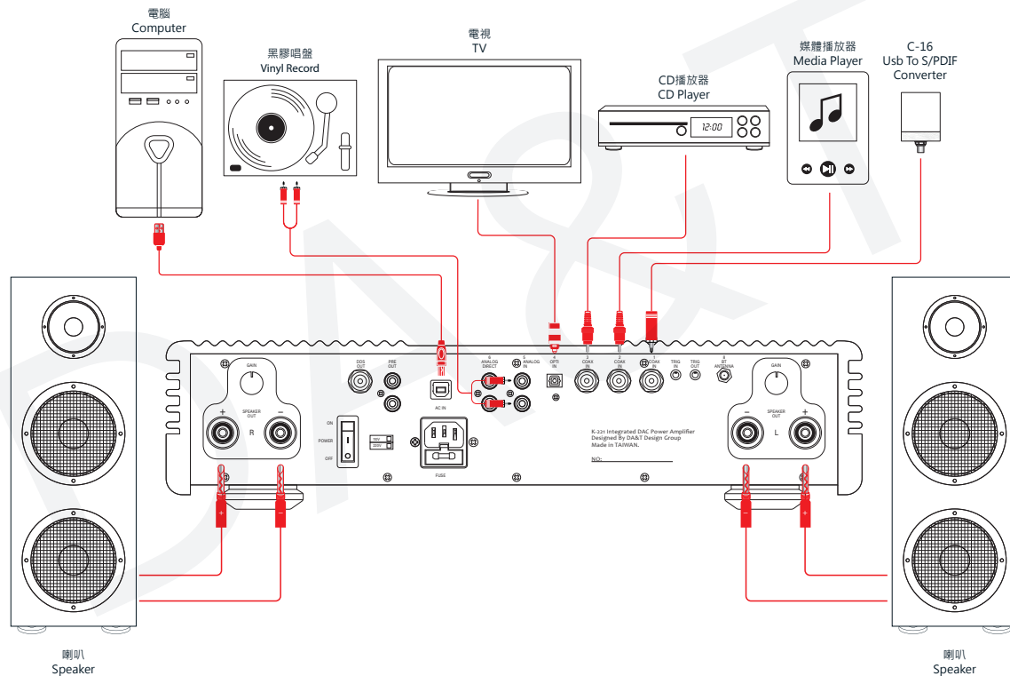
K-221 基本連接圖
