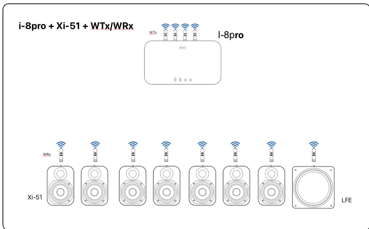
圖九：i-8pro + WTx/WRx + Xi-51x7 + Xi-81
