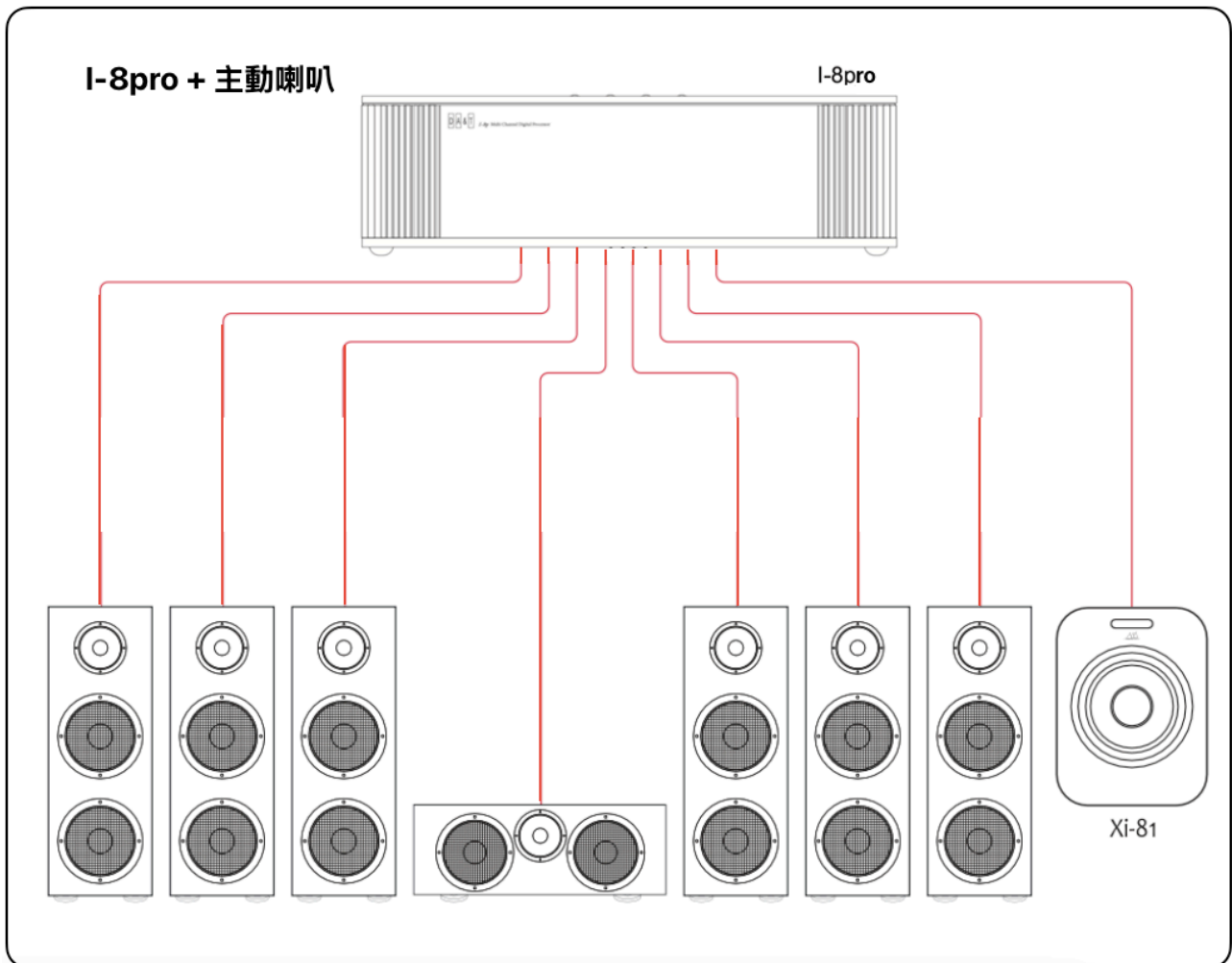
圖六：i-8pro + 類比主動喇叭
