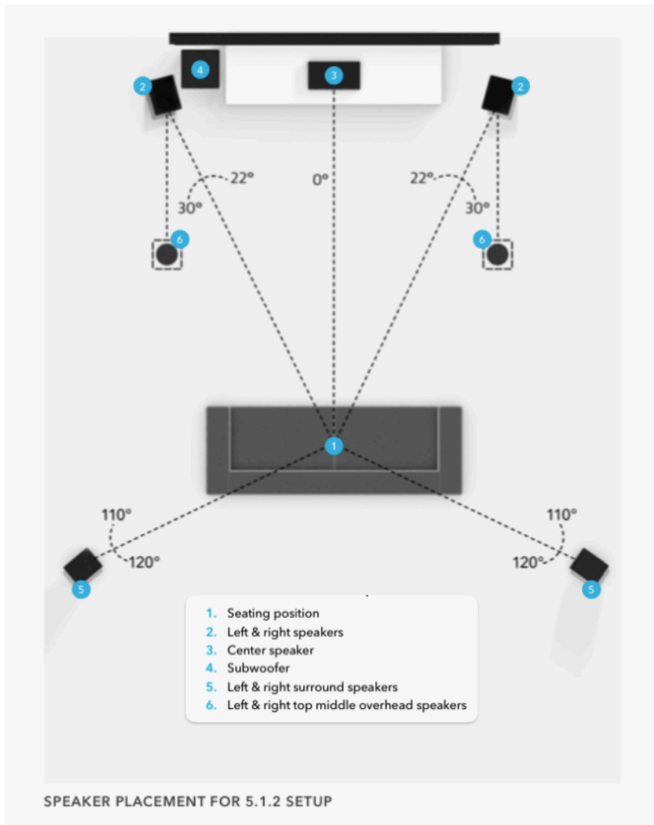
5.1.2 聲道喇叭位置圖（圖一）（圖源取自杜比）
