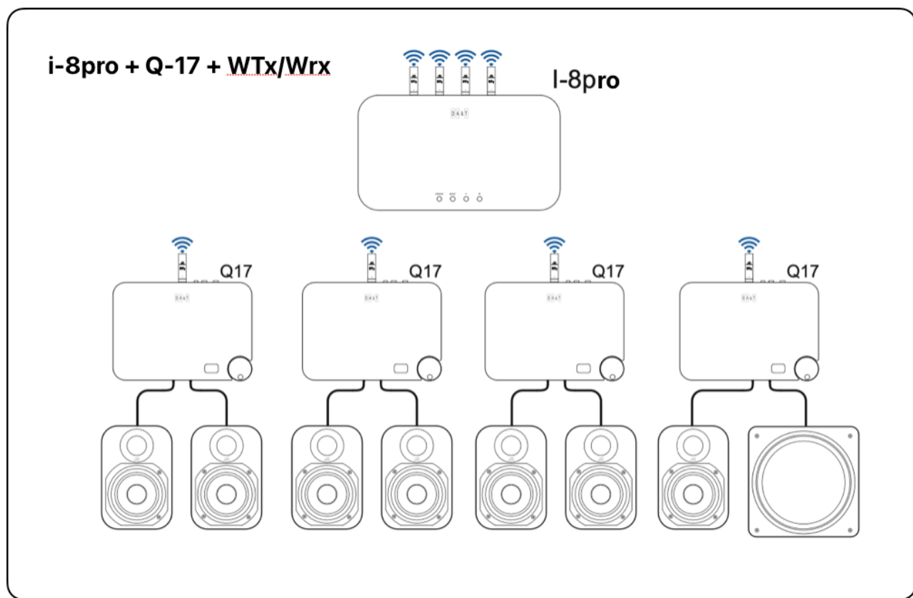
圖八：i-8p + WTx/WRx + Q-17 + 被動喇叭
